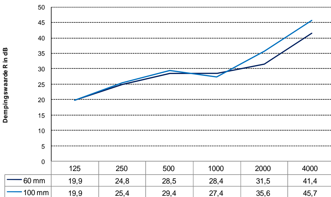
Geluidisolatie
